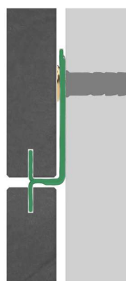
Grapa Intermedia (oculta)
