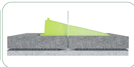
Cuña única en Clip XXL para espesor: de 15 a 25 mm.
