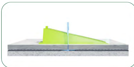
Cuña única en Nox Clip para espesor: de 6 a 14 mm.
