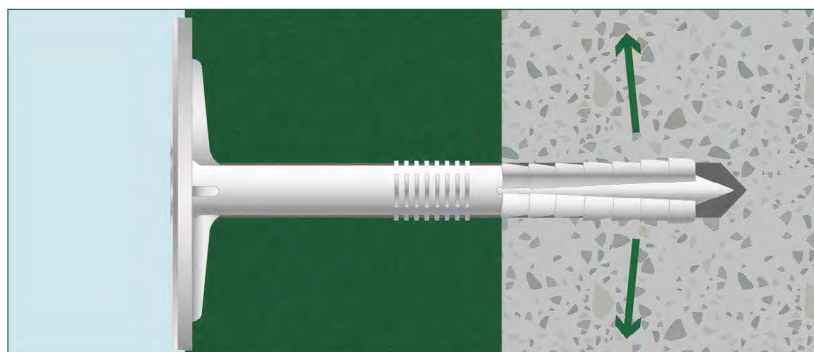
Taco ISO Pro y Eco con clavo de nylon para la colocación de materiales aislantes
