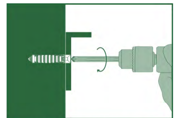
4. Atornillar para expandir el taco.
