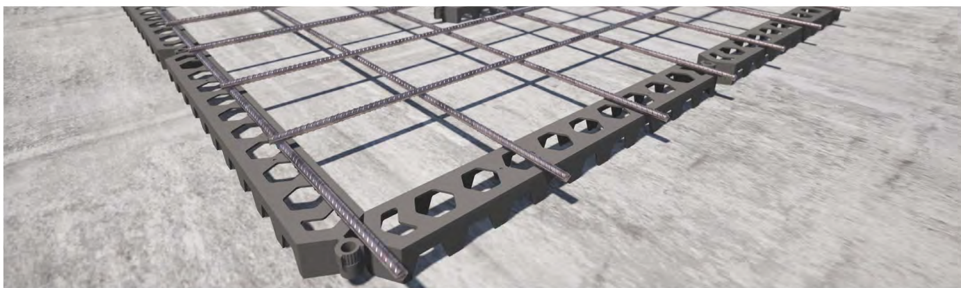
Separador cobra, 40 x 500 mm
