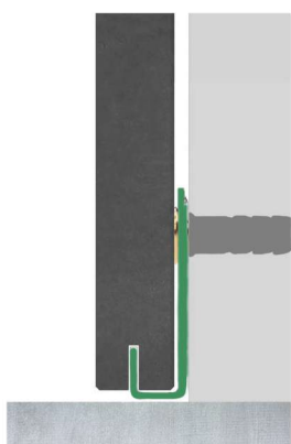
Grapa de Arranque (oculta)
