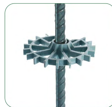
Recomendación colocación en armazón vertical
