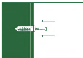
2. Limpiar e insertar el taco
